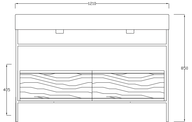
POSIZIONE CASSETTO DESTRO O SINISTRO DRAWER POSITION LEFT OR RIGHT
